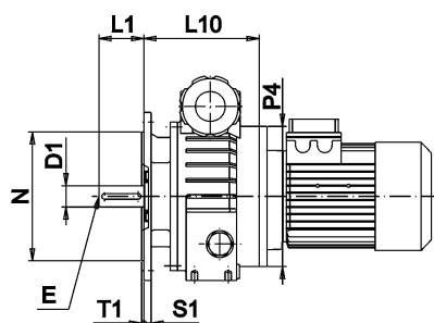
MKFC 30-50 B5
