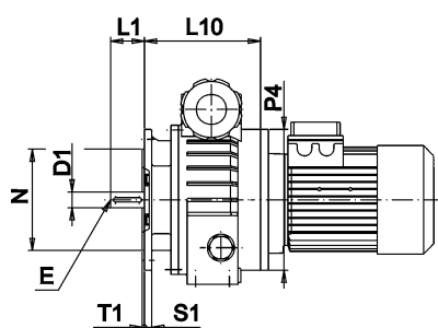
MKFC 30-50 B5
