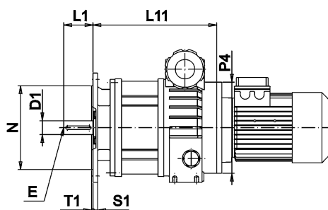
MKDFC 30-50 B5
