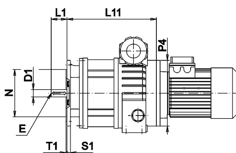
MKDFC 30-50 B5
