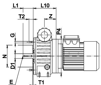
MKFC 20 B5
